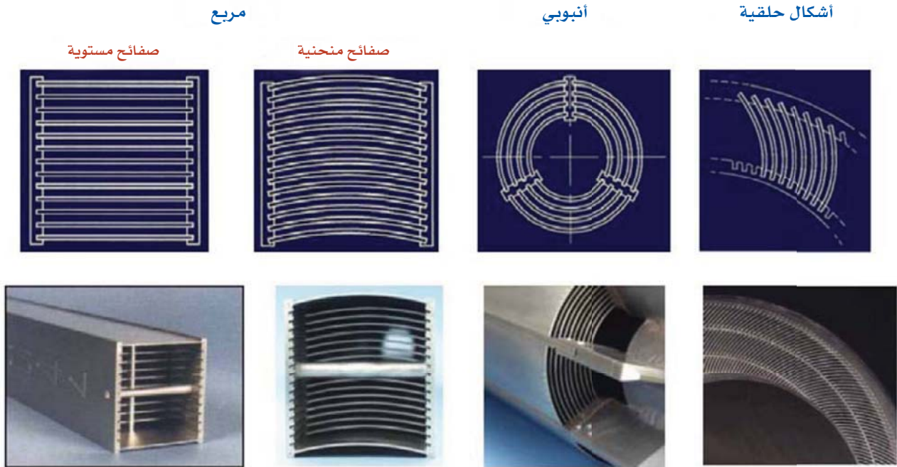
الشكل 1. أمثلة لتصميمات وقود مفاعلات بحثية مختلفة
